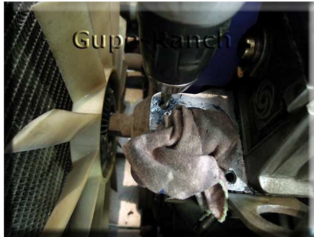
Aufbohren des defekten Gewindes
