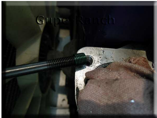
Helicoil-Einsatz mit Spezial-Dorn...
